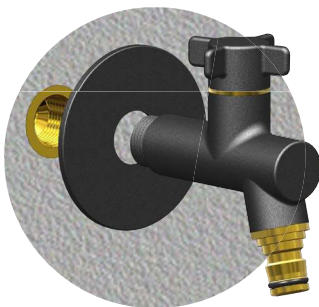
Déformation possible de la rosace de 2 mm maxi par compression lors du vissage du robinet.
