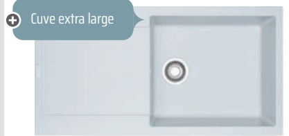
Évier Maris Fraganit, 1 cuve + 1 égouttoir en Blanc arctic Découpe : 950 x 480 mm Hors tout : 970 x 500 mm
