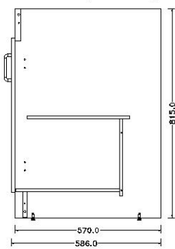
VUE DE DROITE (sans côté droit)
