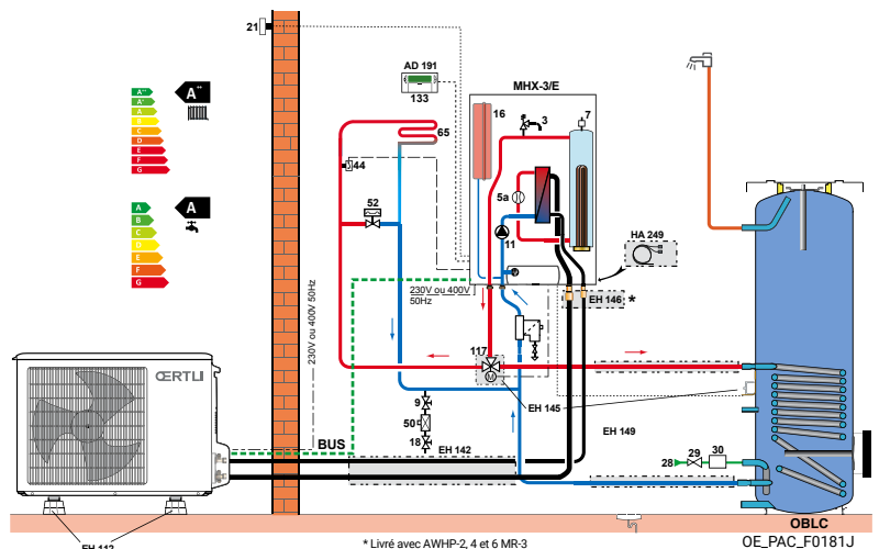
Exemple d'installation, 1 circuit de chauffage avec production d'eau chaude sanitaire
