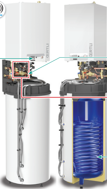
Préparateur e.c.s. en acier vitrifié
