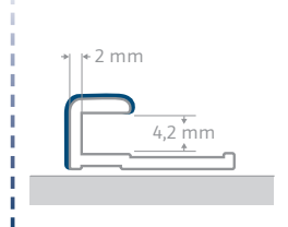
Schéma technique
